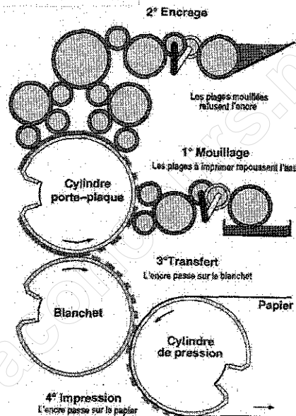
Principe d'une imprimante rotative offset
